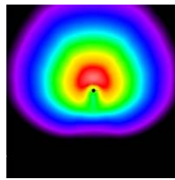
asym. mit haus. Abschirmung Höhe: 4,50m; Fläche: 30m x 30m
